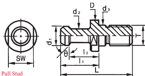
Pull Stud
